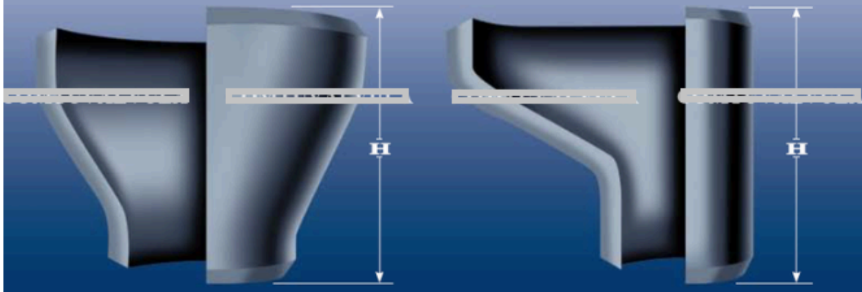
Reducción Concéntrica
